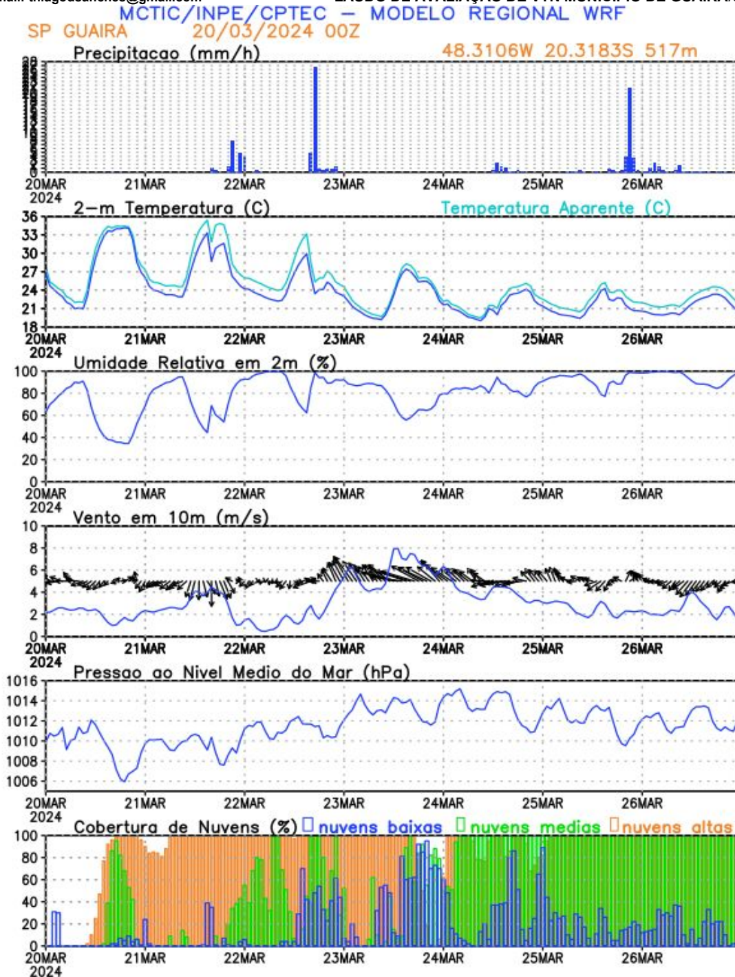
Figura 8. Meteograma do município de Guairá com dados de Precipitação, temperatura, UR, vento em 10 m, PNMM e cobertura de nuvens.
