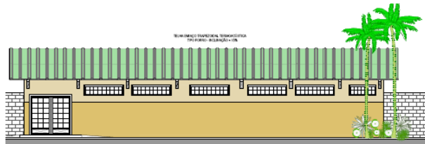
FACHADA FRONTAL
