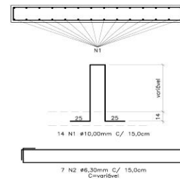
4 DETALHE DO APARELHO DE APOIO DO TANQUE ESCALA 1:25
