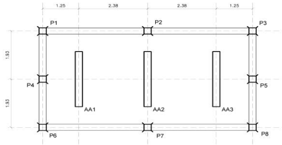
1 LOCAÇÃO ESCALA 1:50
