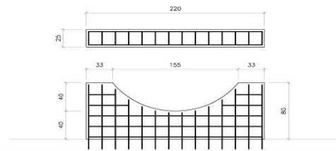
4 DETALHE DO APARELHO DE APOIO DO TANQUE ESCALA 1:25
