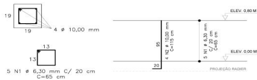
3 DETALHE PILARES S/ESCALA
