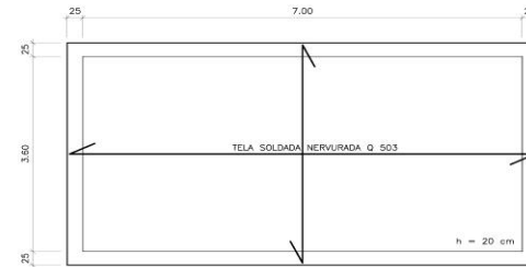
2 RADIER ESCALA 1:50
