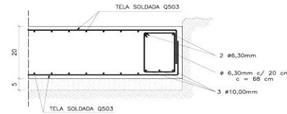
5 DETALHE RADIER - VIGA DE BORDA S/ESCALA
