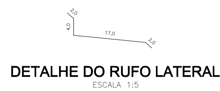
DETALHE DO RUFO PINGADEIRA ESCALA 1:5
