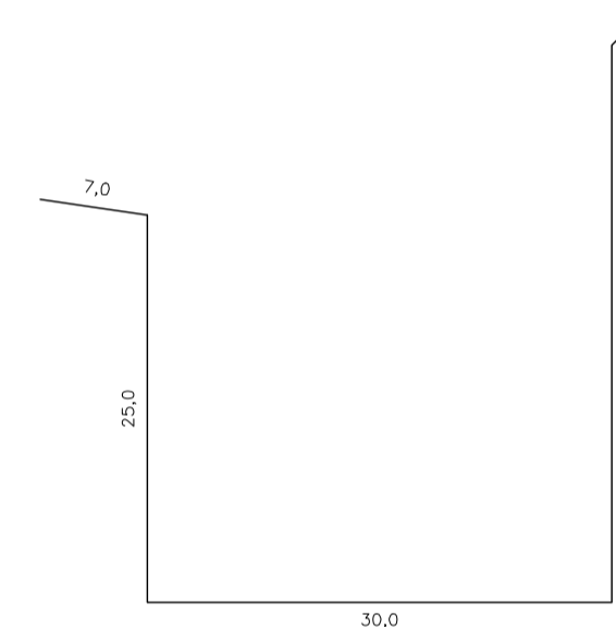
DETALHE DA CALHA ESCALA 1:5
