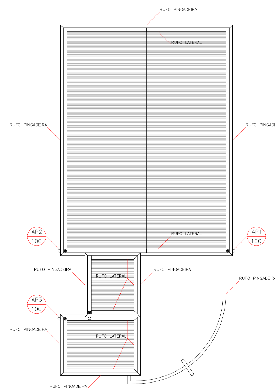
PLANTA DE COBERTURA ESCALA 1:100
