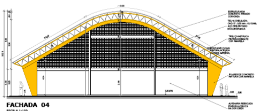
FACHADA 04 ESCALA 1:100
