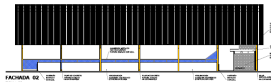
FACHADA 02 ESCALA 1:100
