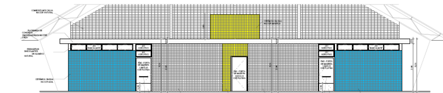
VESTIÁRIO: VISTA E - FACHADA FRONTAL
