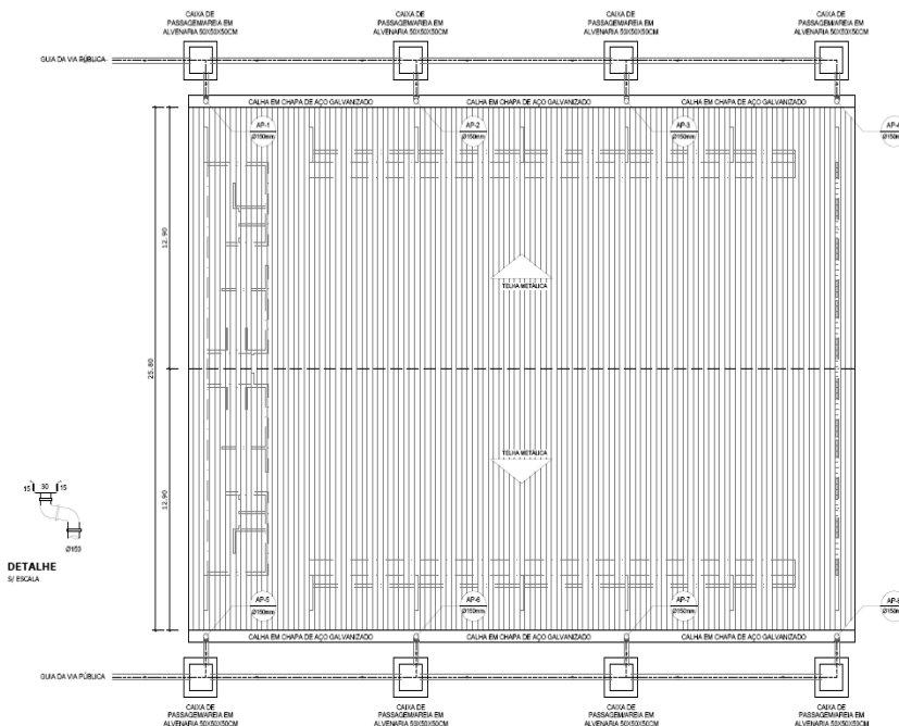
PLANTA DE COBERTURA ESCALA 1:150
