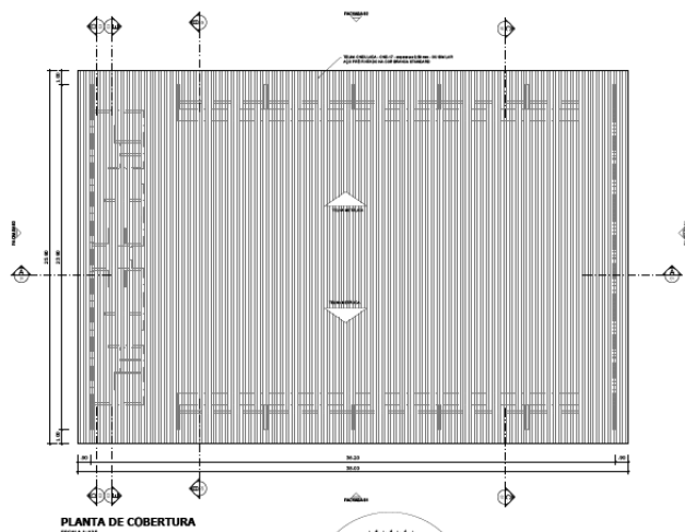
PLANTA DE COBERTURA ESCALA 1:100
