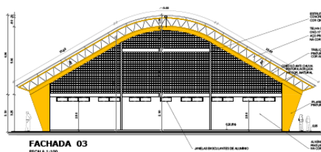
FACHADA 03 ESCALA 1:100
