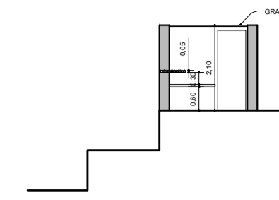
CORTE - CABINES
