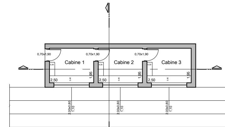
PLANTA - CABINES
