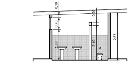
CORTE - BAR/BHOS 2
