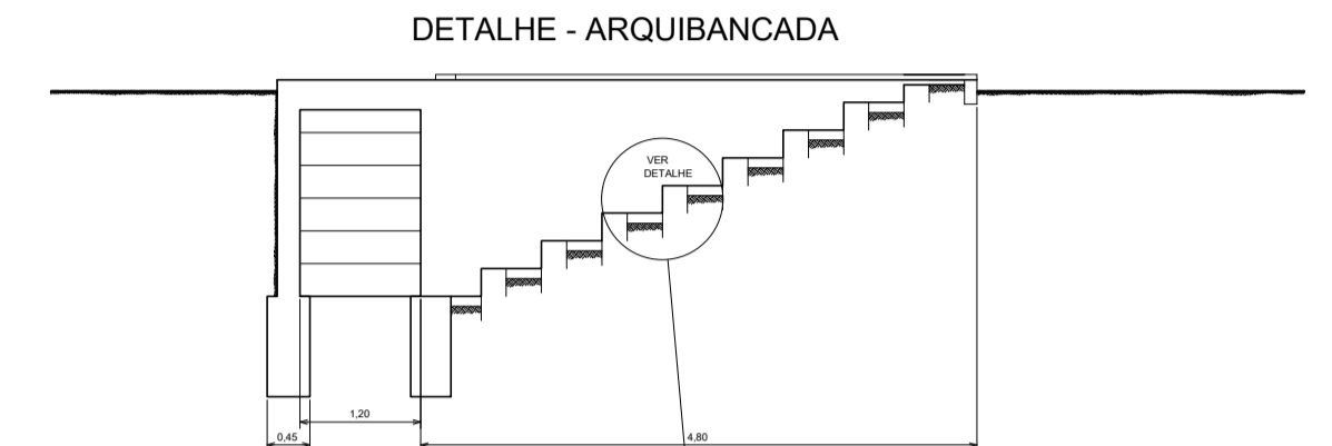
DETALHE - ARQUIBANCADA
