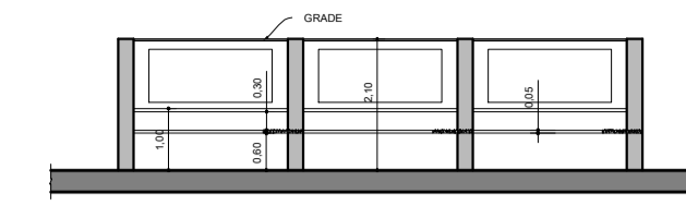
CORTE - CABINES
