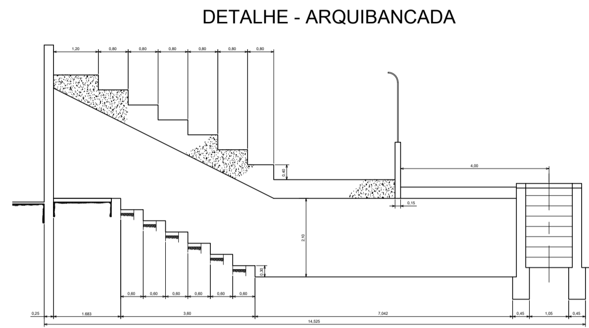
DETALHE - ARQUIBANCADA
