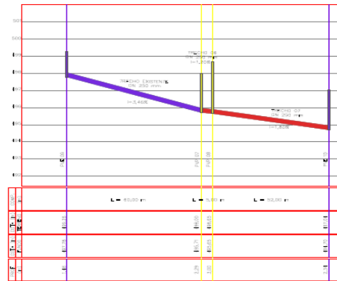
PERFIL - TRECHO 06 E 07 Escala: 1/500
