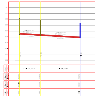
PERFIL - TIE/H05 01 E 02 E10-L1 - 1/500
