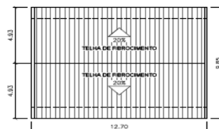
2 COBERTURA ESCALA 1:150
