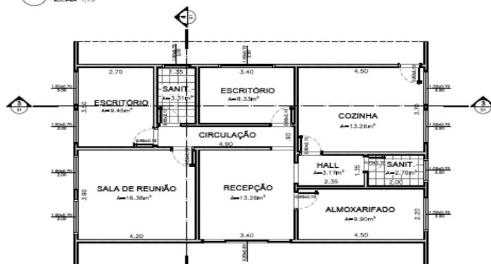
1 PLANTA BAIXA ESCALA 1:75
