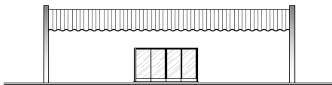
5 FACHADA ESCALA 1:75
