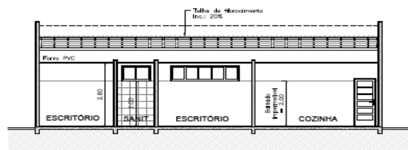
3 CORTE LONGITUDINAL ESCALA 1:75
