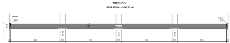
DETALHE DA GEOMETRIA DA RUA 28 ENTRE AS AV. 36 E AV. 27 ESC. 1:500
