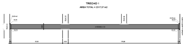
DETALHE DA GEOMETRIA DA AV. 35 ENTRE AS RUAS 38 E AV. JOSÉ FLORES ESC. 1:500
