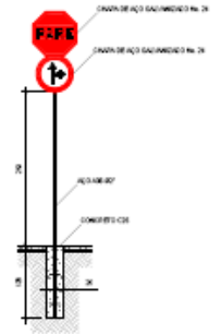
DETALHE DA SINALIZAÇÃO VERTICAL ESC. 1:40
