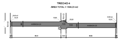
DETALHE DA GEOMETRIA DA AV. 33 ENTRE AS RUAS 20 E RUA 24 ESC. 1:500
