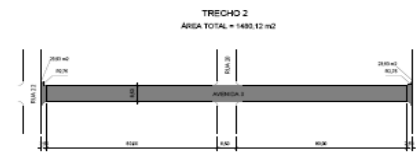
DETALHE DA GEOMETRIA DA AV. 3 ENTRE AS RUAS 22 E RUA 18 ESC. 1:500
