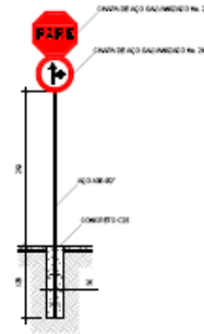
DETALHE DA SINALIZAÇÃO VERTICAL ESC. 1:40
