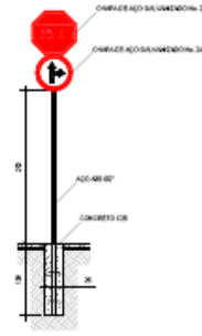
DETALHE DA SINALIZAÇÃO VERTICAL ESC. 1:40
