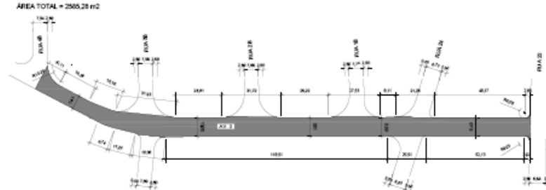
DETALHE DA GEOMETRIA DA AV. 3 ENTRE AS R. 4B E R. 22 ESC. 1:1000
