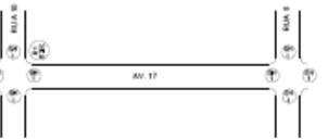
DETALHE DA GEOMETRIA DA AV. 17 ENTRE AS R. 8 E R. 10 ESC. 1:100
