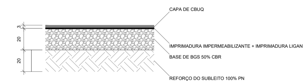
DETALHE DA PAVIMENTAÇÃO ESC. 1:20
