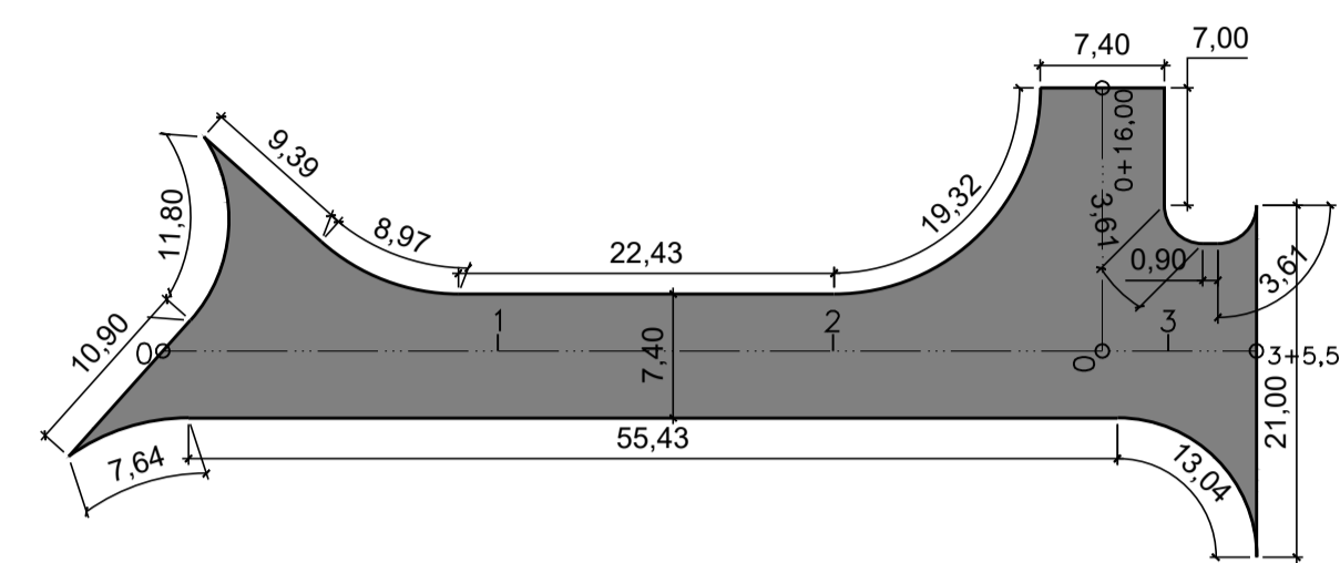
GEOMETRIA - RUA "DR. LUIZ ROBERTO BONJORNO" ÁREA TOTAL = 686,96 m 2 ESCALA 1 : 500
