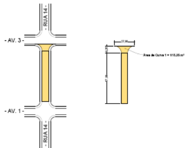
DETALHE DO RECAPEAMENTO ESC. 1:20
