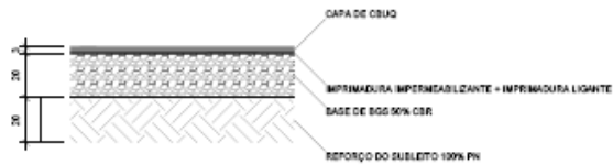
DETALHE DA PAVIMENTAÇÃO ESC. 1:20
