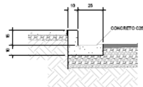
DETALHE DA GUIA E SARJETA ESC. 1:40
