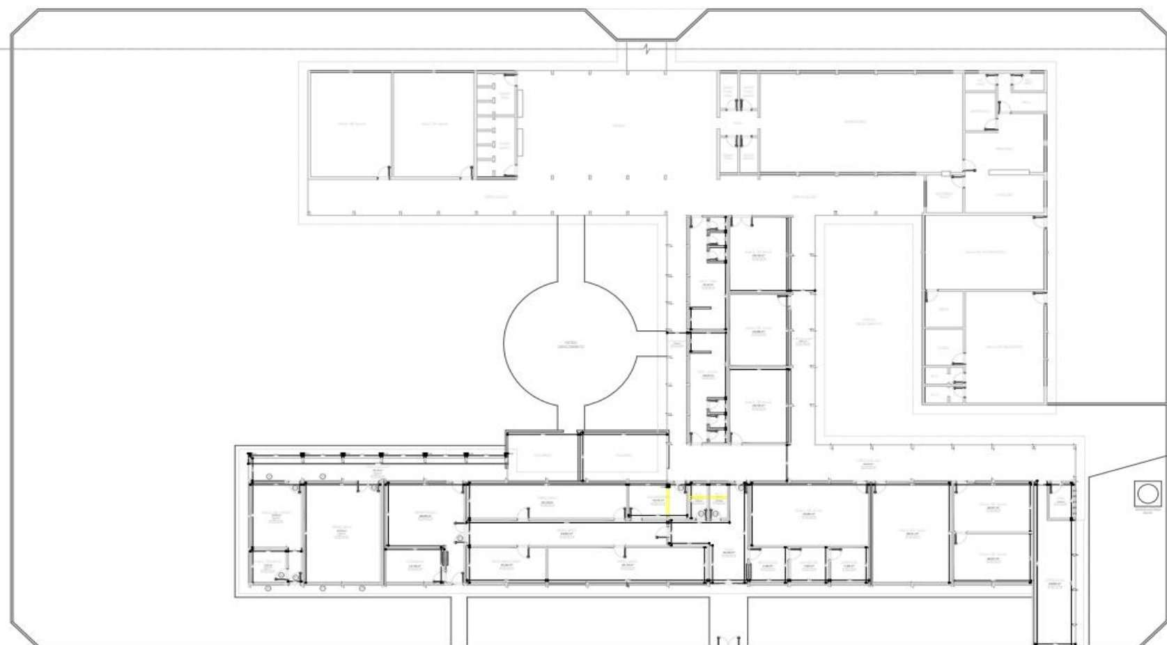
PLANTA BAIXA ESCALA 1:100
