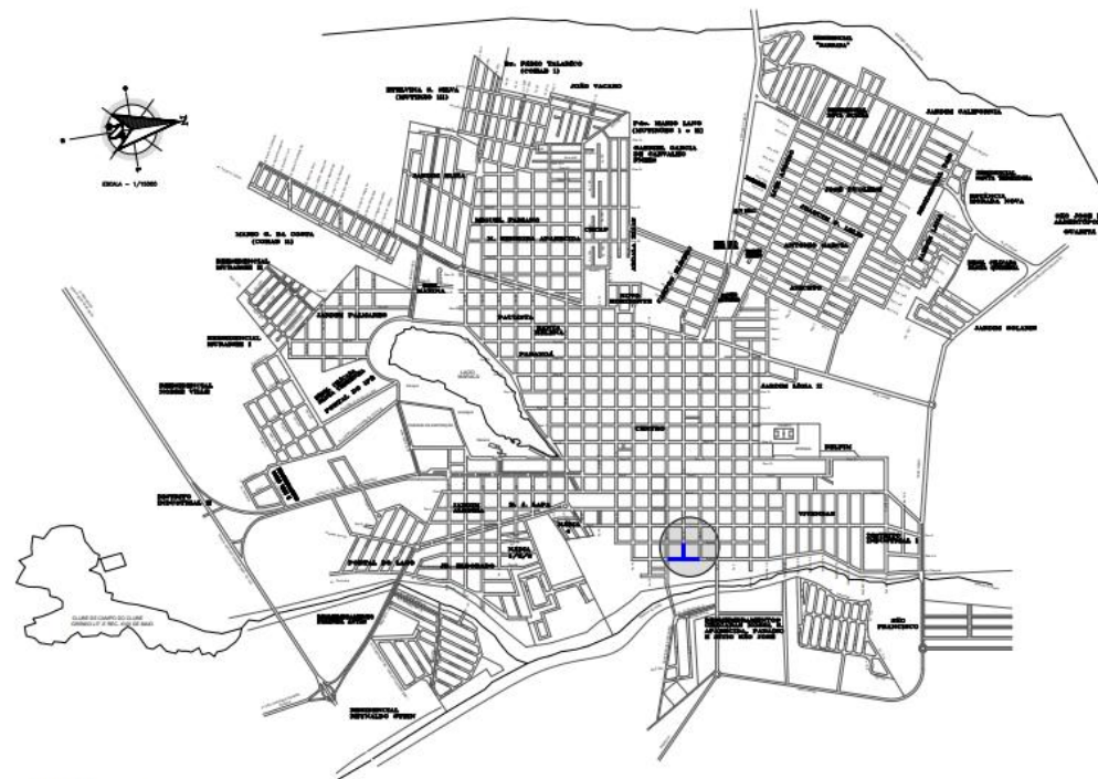
PLANTA DE LOCAÇÃO ESC. 1:10000
