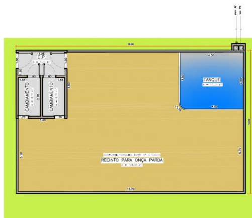
1 PLANTA BAIXA ESCALA 1:100
