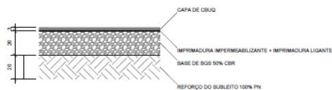
DETALHE DA PAVIMENTAÇÃO ESC. 1:20
