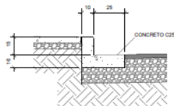
DETALHE DA GUIA E SARJETA ESC. 1:40
